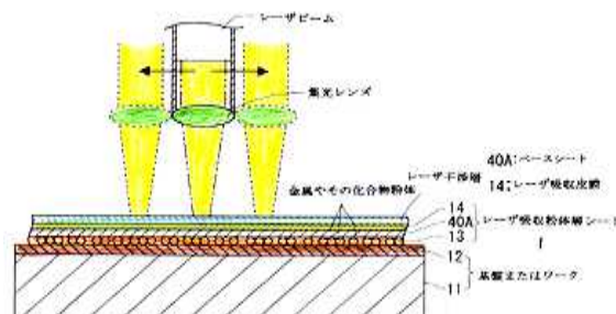
図1 特殊レーザピーニング原理図
