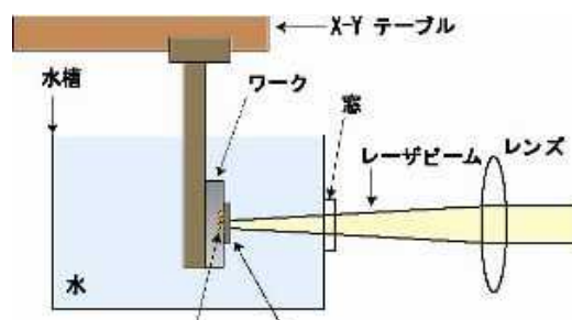
図2 水中でピストンにピーニング
